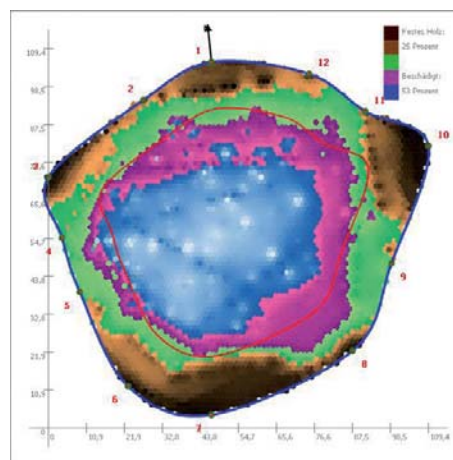
Die Holzqualität unter der Rinde machen wir mit Ultraschall sichtbar. Der Baumbesitzer sieht sofort, welche Bäume gefährdet sind.
